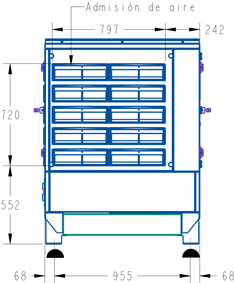
VISTA LATERAL
