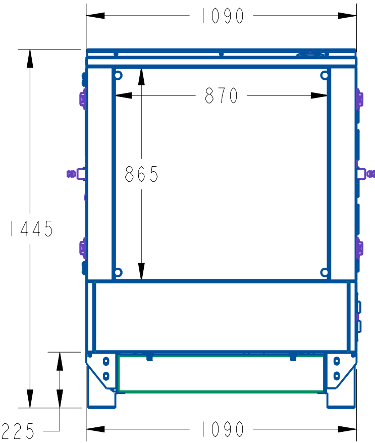
VISTA LATERAL
