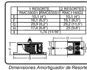
Dimensiones Amortiguador de Resorte
