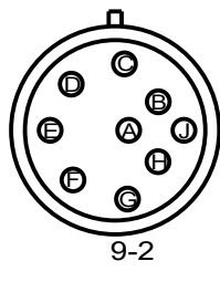
CONECTORES DEUTSCH
