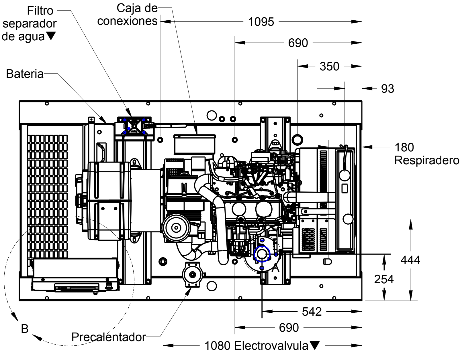
VISTA SUPERIOR
