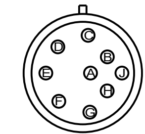
CONECTOR DEUTSCH
