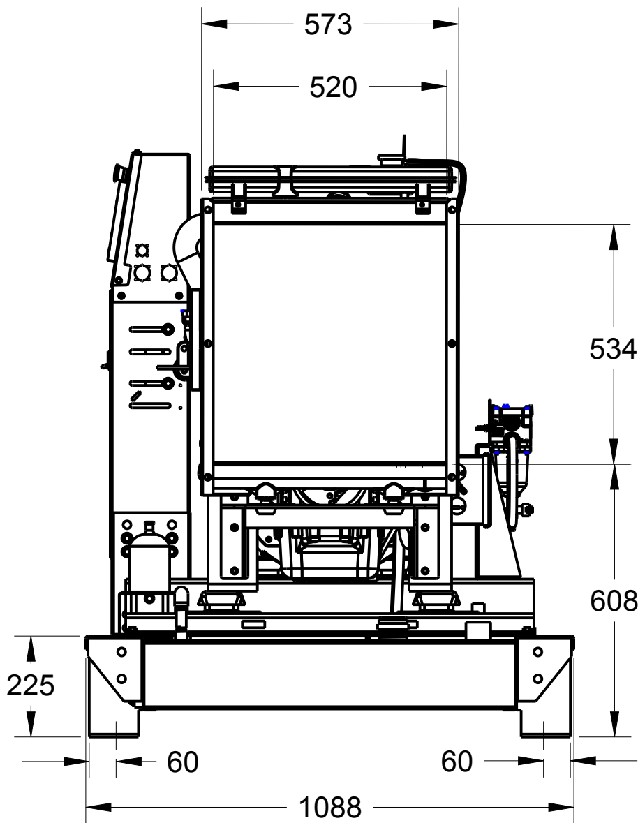
VISTA LATERAL
